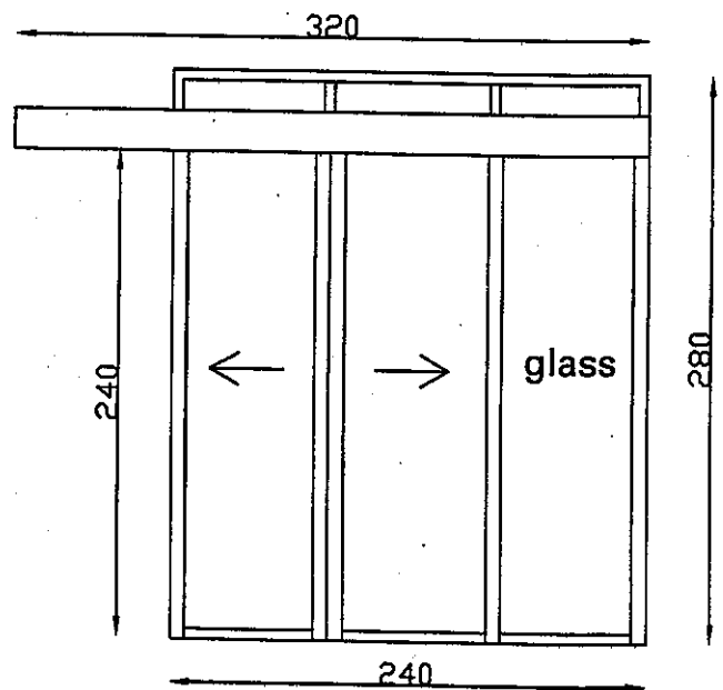
درب اتوماتیک اسلایدینگ دوطرف بازشو دفتر فنی قدرت
