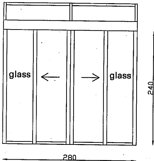
درب اتوماتیک اسلایدینگ دوطرف بازشو دفتر فنی قدرت
